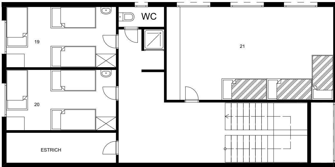
3.OBERGESCHOSS MST. 1:200
