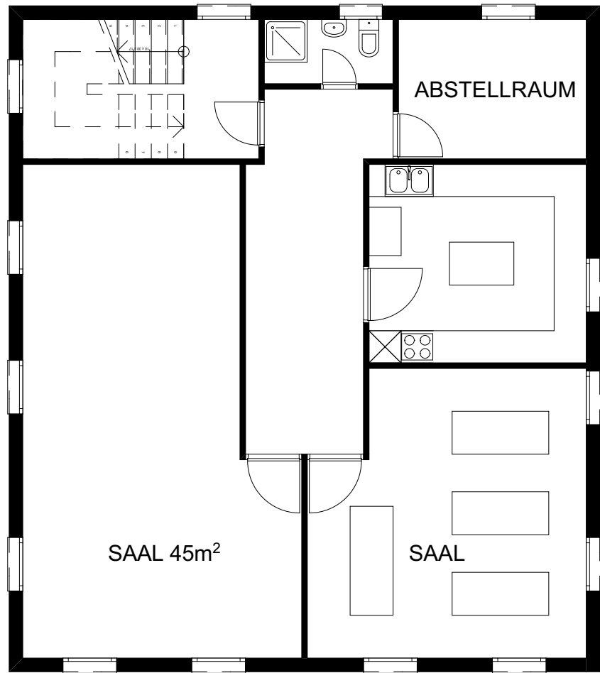
1. OBERGESCHOSS 1:100
