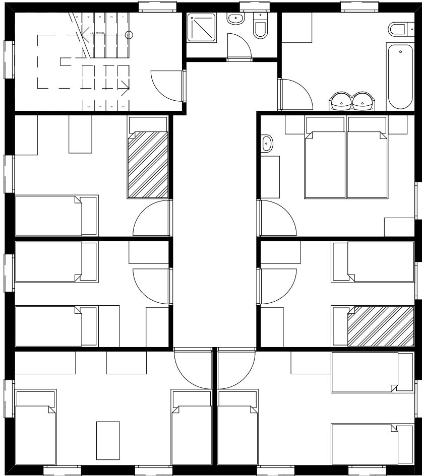
2. OBERGESCHOSS 1:100
