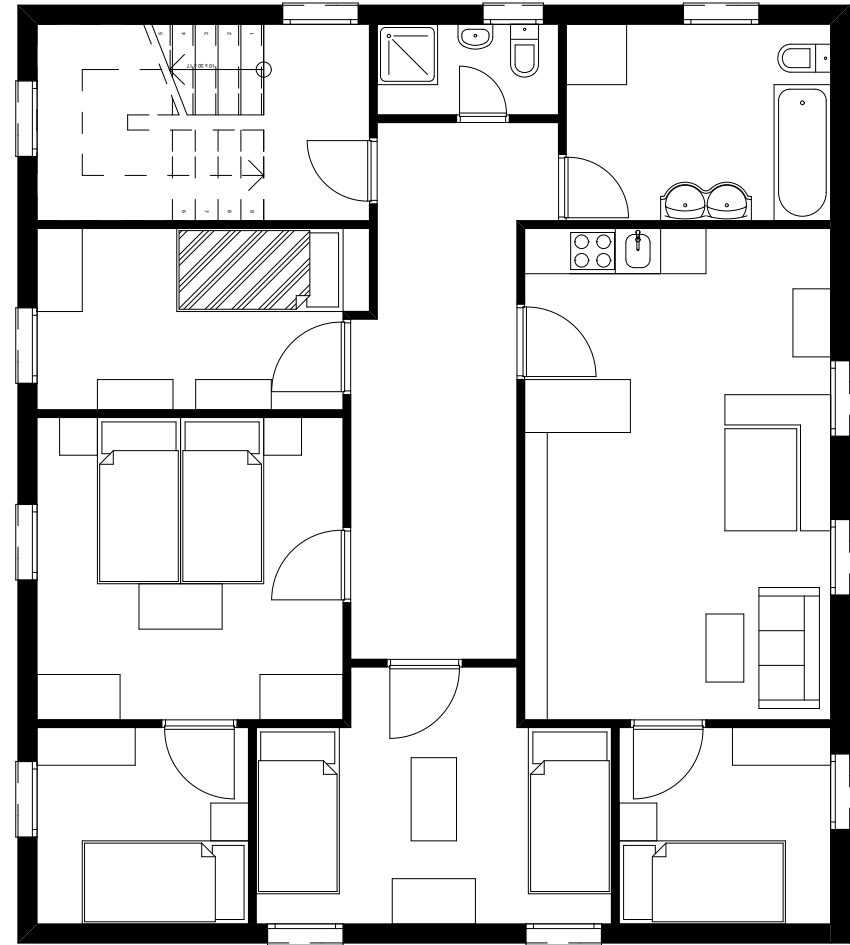
3. OBERGESCHOSS 1:100
