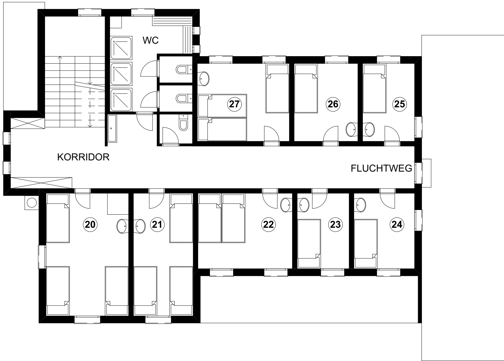
2.OBERGESCHOSS MST. 1:100
